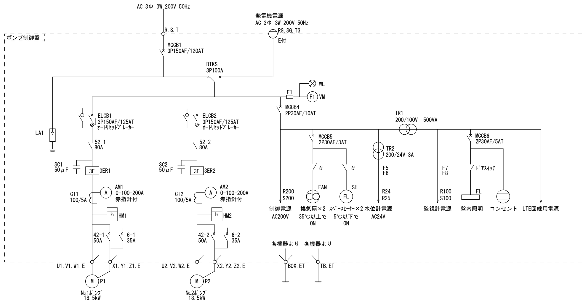
単線結線図
