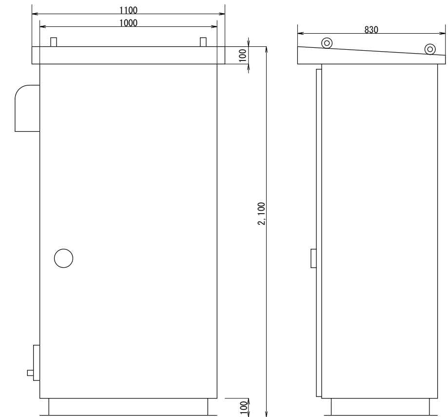
正面図
