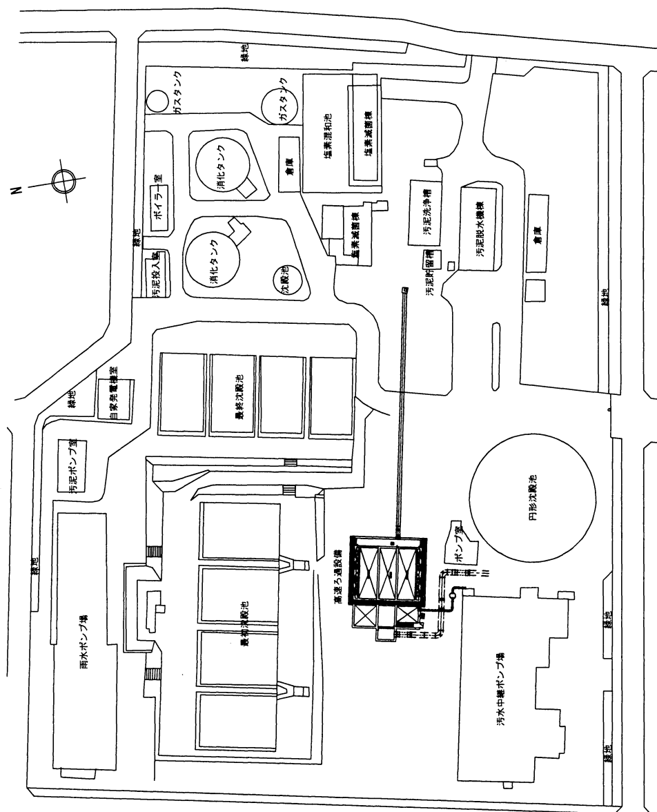
住宅ポンプ場平面図
